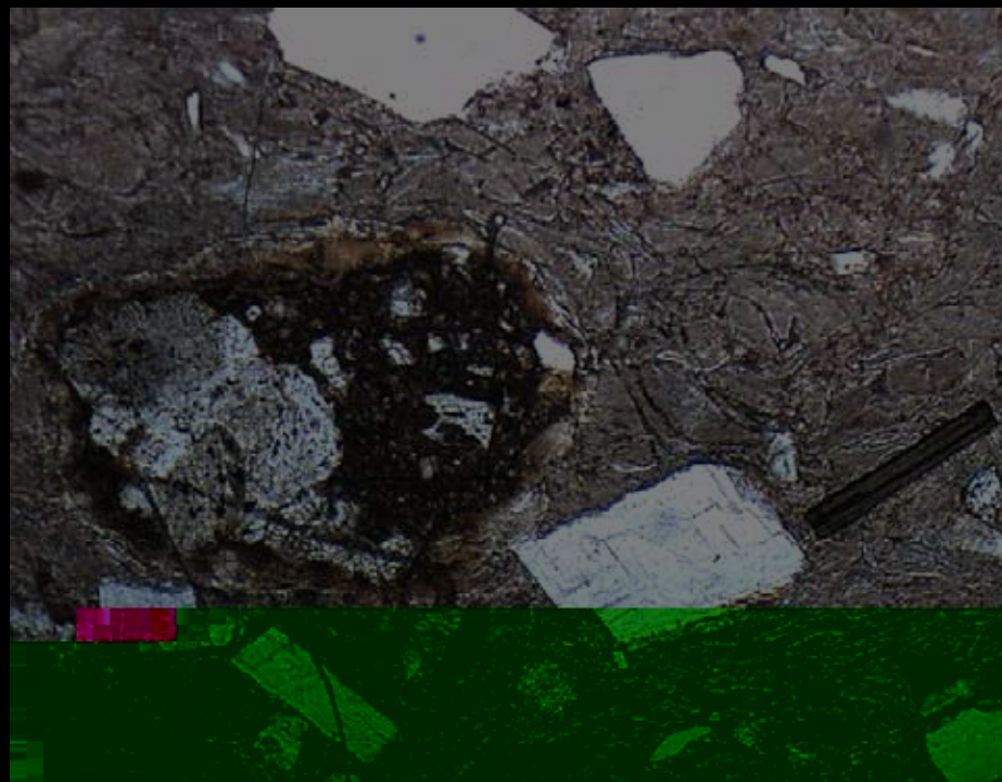
凝灰岩刚性岩屑
